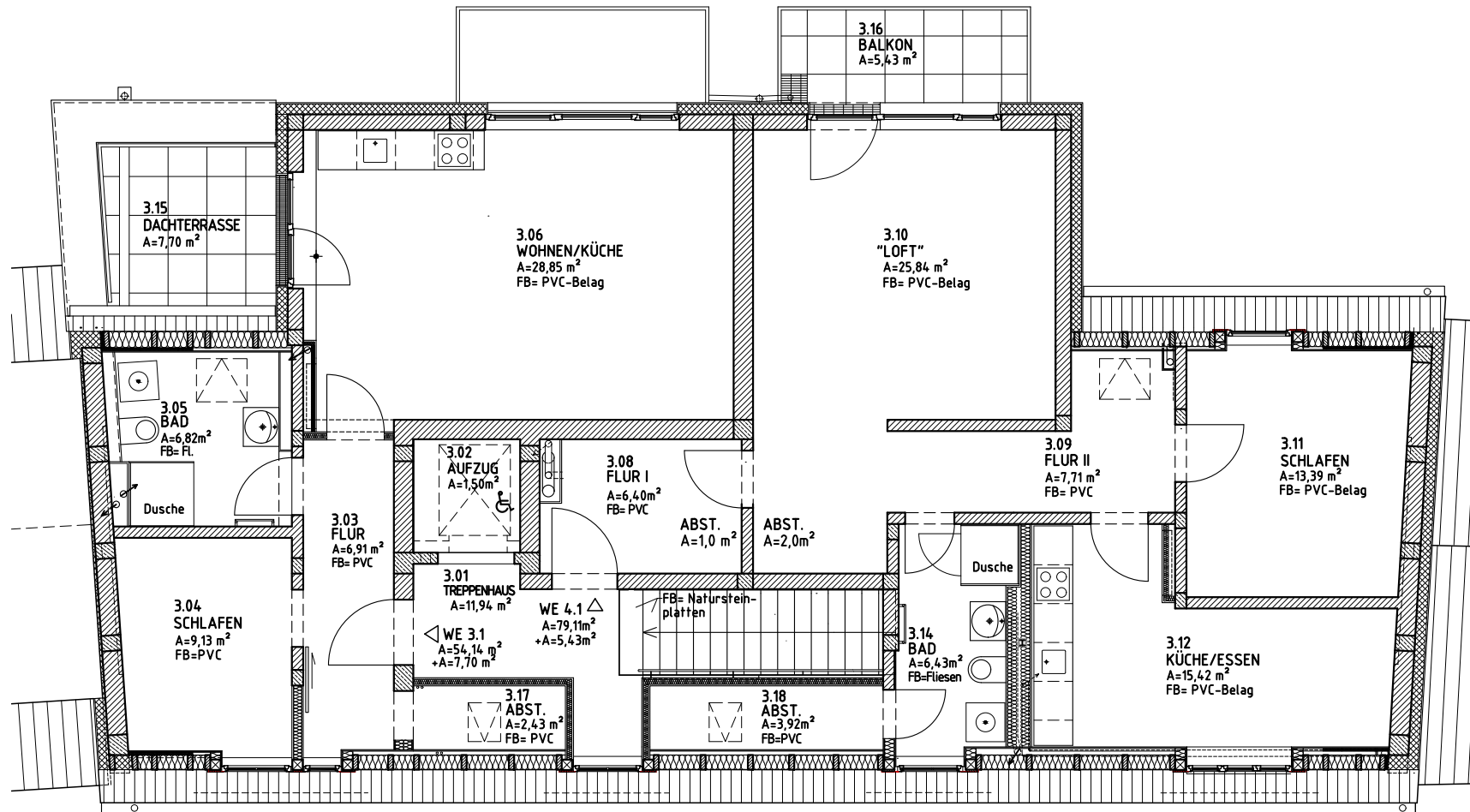
DACHGESCHOSS
